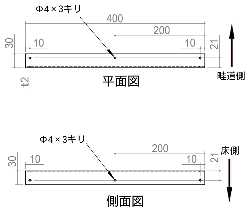
堰枠保護用アンクル加工図 A6063 ( 30 × 30 × t2 × 400mm )
